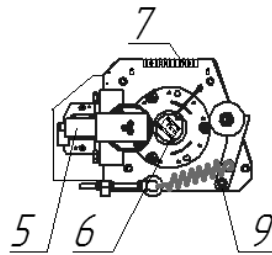
А (крышка не показана)
