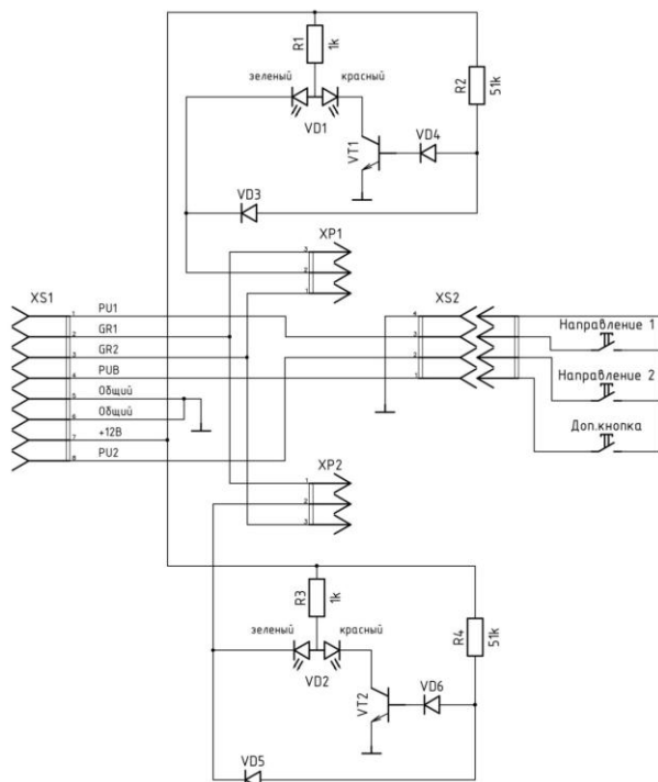
Схема электрическая принципиальная пульты дистанционного управления П2П-0-0Г
