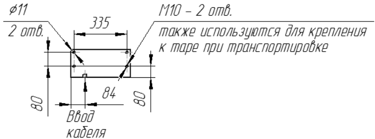
Габаритные и установочные размеры турникета «Ростов-Дон Т8М1»
